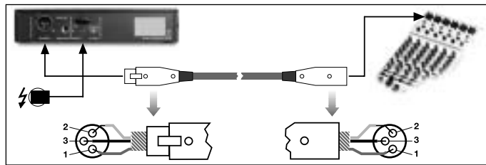
Fig. 3: Collegamento del ricevitore ad un ingresso simmetrico sul mixer
