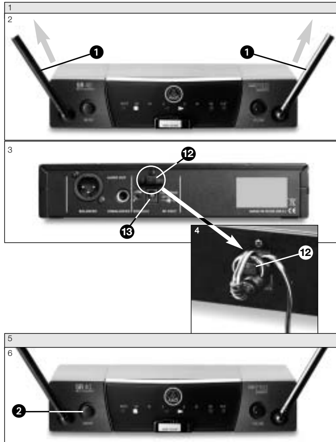
Abb. 5: Netzanschluss
