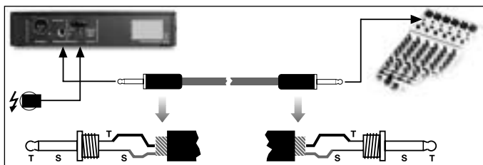
Fig. 4: Conectar o receptor a uma entrada desbalanceada na mesa de mixagem
