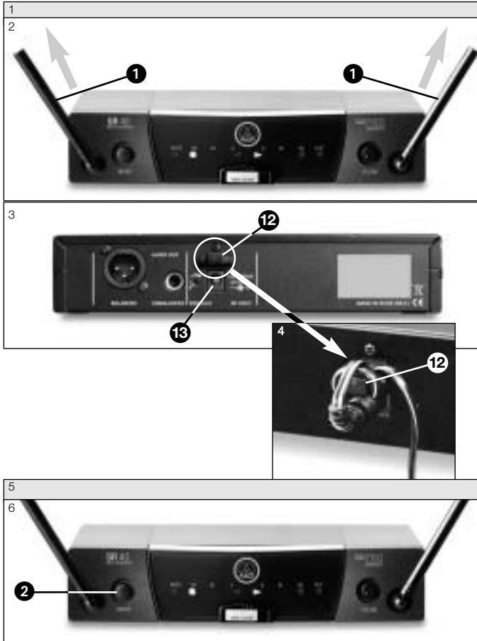
Fig. 5: Antenna - dispositivo antitrazione - attivazione
