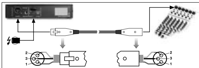
Fig. 3: Conectar o receptor a uma entrada balanceada na mesa de mixagem
