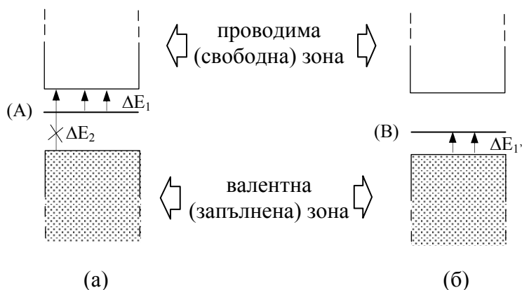
фиг.4. Два механизма за външна проводимост на полупроводниците.
